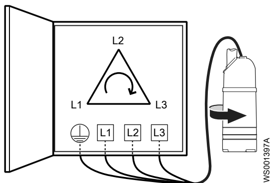
Figura 3: Reacción de arranque
