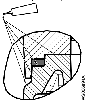
Figura 4: Ejemplo de superficies adyacentes a juntas tóricas
