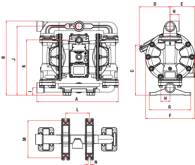
DIMENSIONES (mm)
