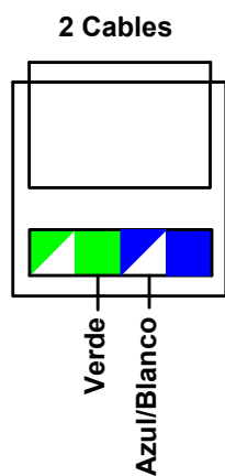
CONEXIÓN PARA TELÉFONOS CON 2 CABLES
