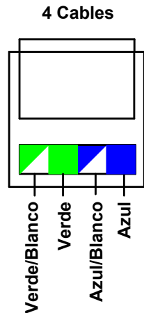
CONEXIÓN PARA TELÉFONOS CON 4 CABLES
