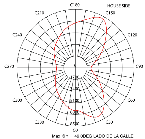
DIAGRAMA DE DISTRIBUCIÓN DE INTENSIDAD MÁXIMA DE LA SUPERFICIE DEL CONO
