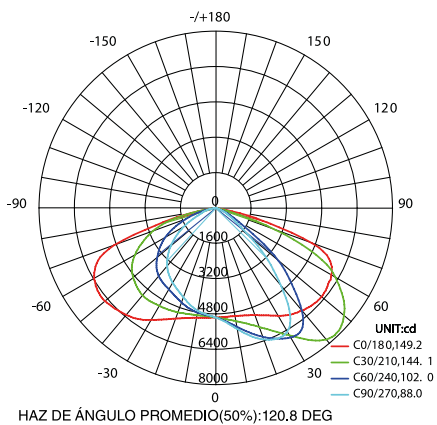
DIAGRAMA DE ISOCANDELA
