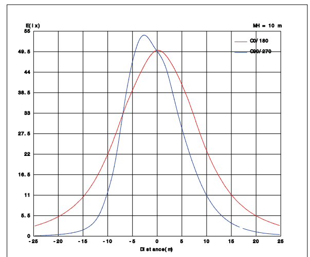
CURVA DE ILUMINANCIA PLANA
