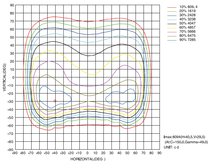
DIAGRAMA DE ISOCANDELA
