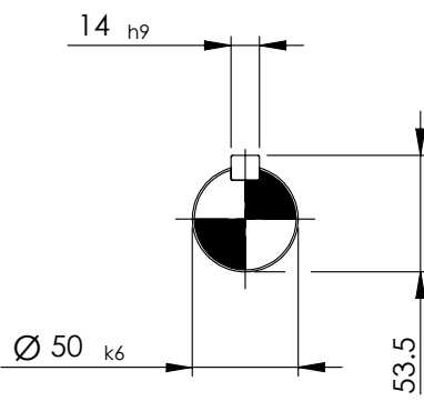
Detalhe eixo de saída Output Shaft Detail Detalle eje de salida (Sem escala/no scale/sin escala)
