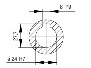
Detalhe entrada do motor Shaft motor detail Detalle entrada motor (Sem escala/no scale/sin escala)
